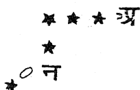
चित्र ४—मृगशीर्ष नीहारिका
